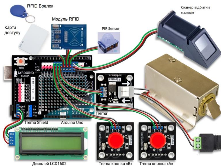
Рисунок 1. – Система контролю доступу на базі Arduino
