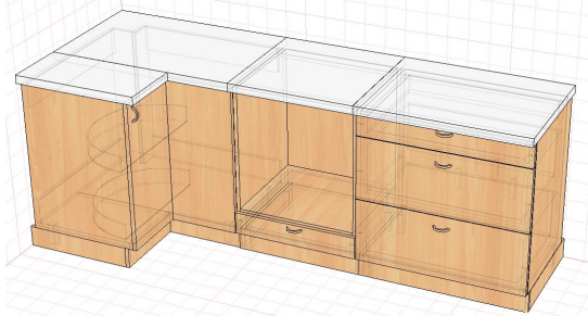
Рис. 5. Проектування нижньої частини кухонного набору з готових модулів
