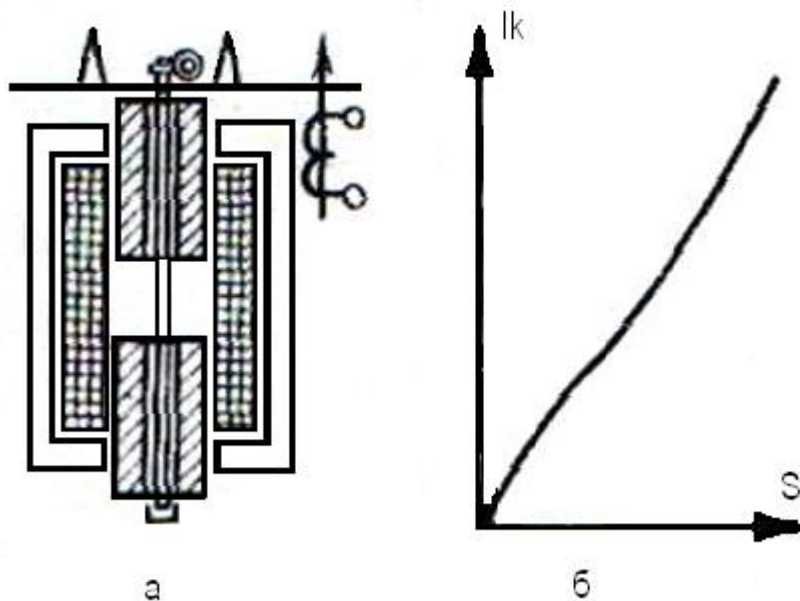
Рисунок 1.2 - Плунжерний ДР: а – загальний вигляд; б – залежність струму компенсації від фактору регулювання
