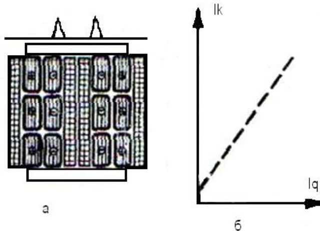
Рисунок 1.4 - ДР зі змушеним поперечним підмагнічуванням: а – загальний вигляд; б – залежність струму компенсації від фактору регулювання
