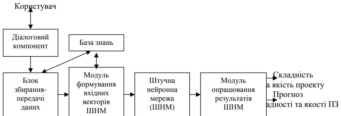
Рис.2. Структурна схема ІСОП
