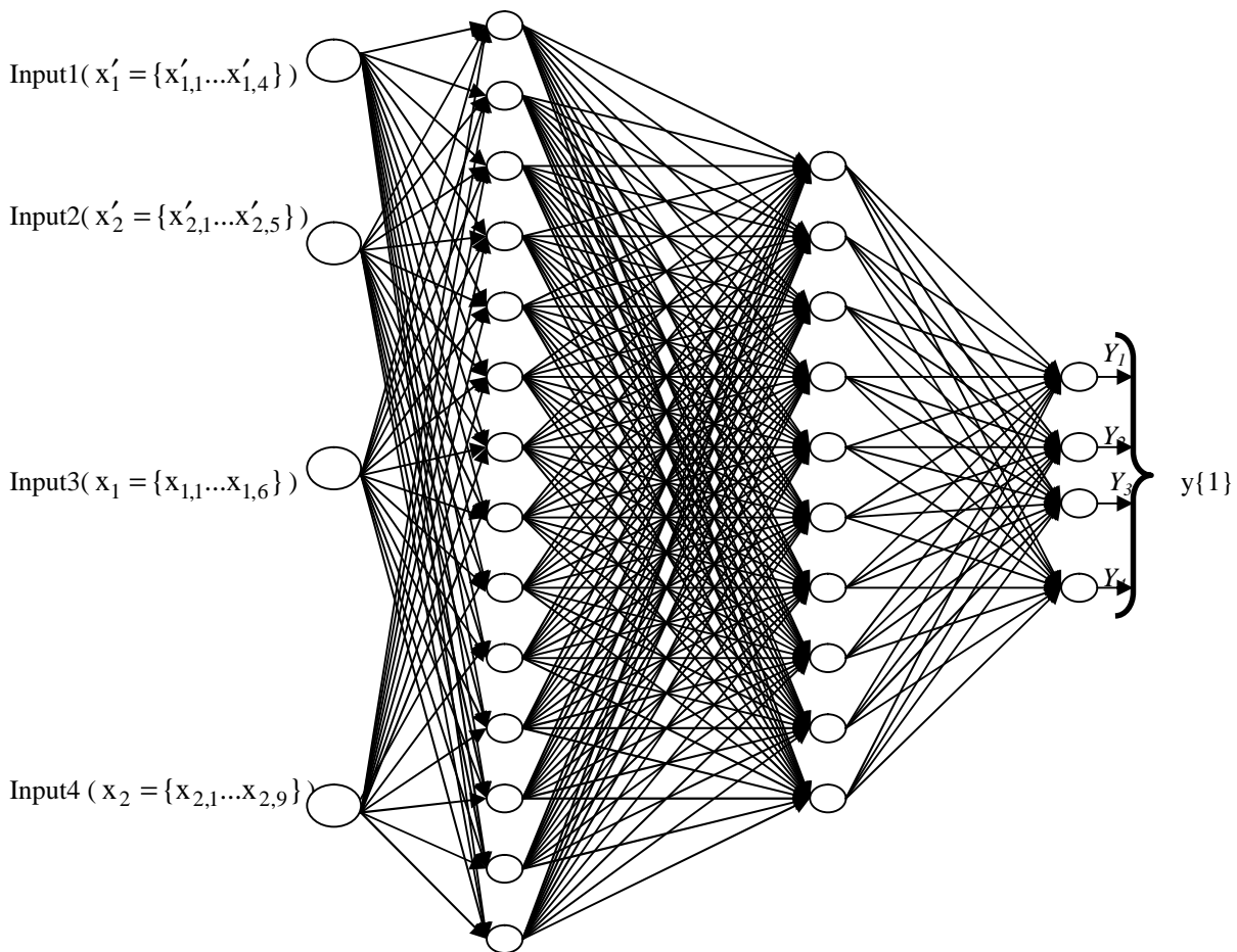
Рис.3. Архітектура ШНМ
