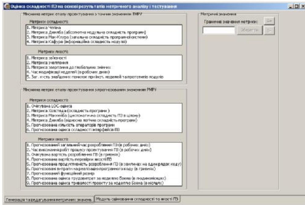
Рис.4. Перше інтерфейсне вікно системи ІСОП (довідкове)
